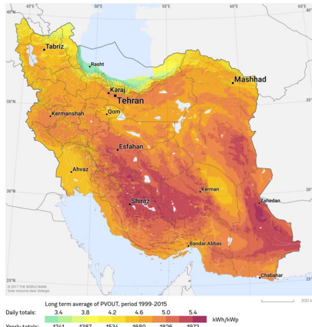
شکل ۱- نقشه میانگین روزانه و سالانه تولید برق فوتولتائیک در ایران
