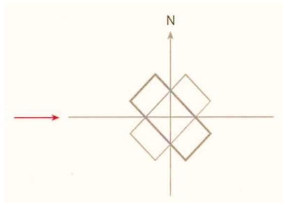
شکل B: جهت قرار گیری مناسب برای استفاده از باد های شرقی یا غربی. (هاشمی ، ۱۳۹۰) (کسمایی ، صفحه ۶۸، ۲۰۰۳)
