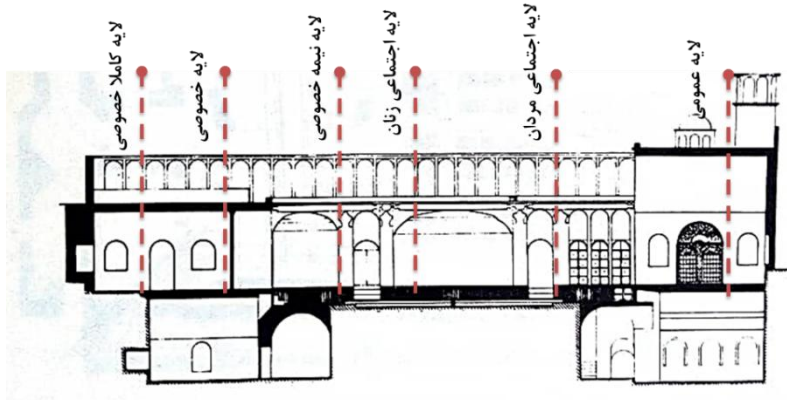
تصویر ۲: لایه های حریم در خانه رسولیان یزد (برگرفته از: معماریان، ۱۳۷۳، ۳۱۷) تحلیل نگارندگان
