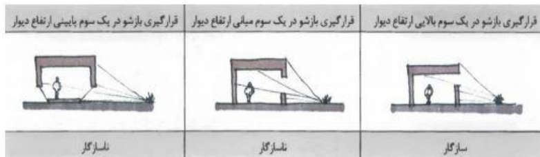
شکل ۱۸_ محل قرارگیری بازشو نسبت به ارتفاع دیوار، ماخذ: (جهانگیری، ۱۳۹۴)
