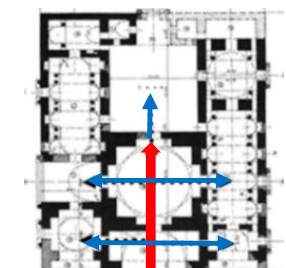
شکل ۱۶- الگوی روابط فضایی کاخ سروستان (مأخذ: Pope, 1933: 63)
