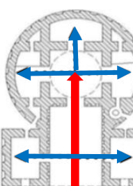
شکل ۱۵- الگوی سازماندهی فضایی سطح سوم قلعه دختر (مأخذ: ارژمند و اعتمادی پور، ۱۳۹۲: ۵۳)
