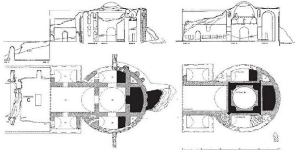
شکل ۸- نقشه و مقطع بنای قلعه دختر (مأخذ: huff, 2005: 389)
