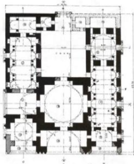
شکل ۲۴- پلان و برش عمودی کاخ سروستان (مأخذ: Pope, 1933:63)
