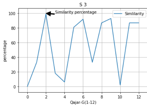
شکل ۱۳. تشابه سنجی پلان شماره ۳ صفوی با ۱۲ پلان قاجار.
